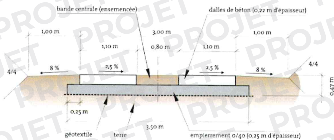
Coupe de principe
