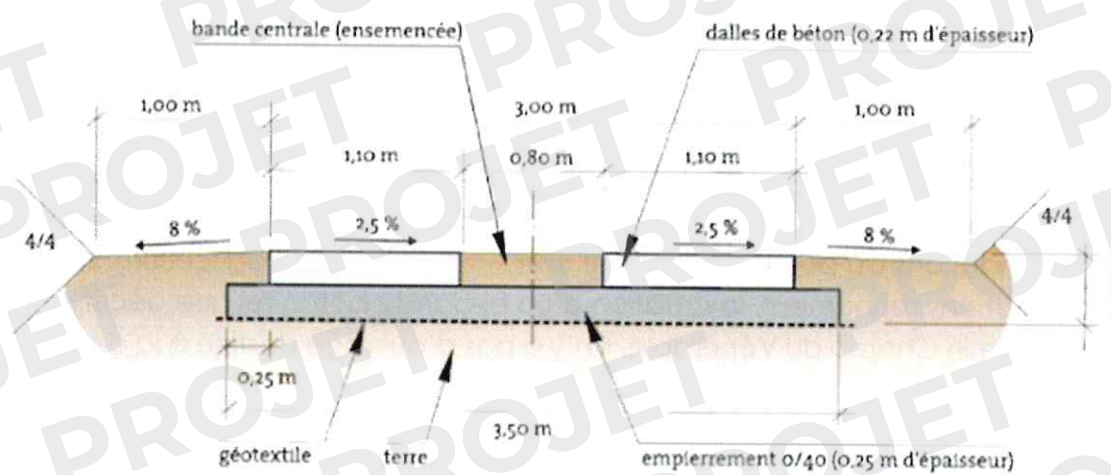
Coupe de principe
